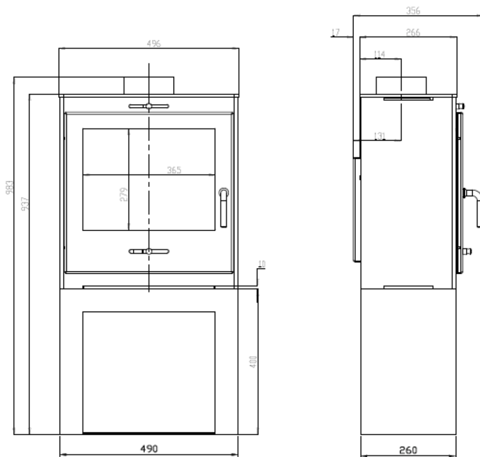
Technický výkres hede 1D:
